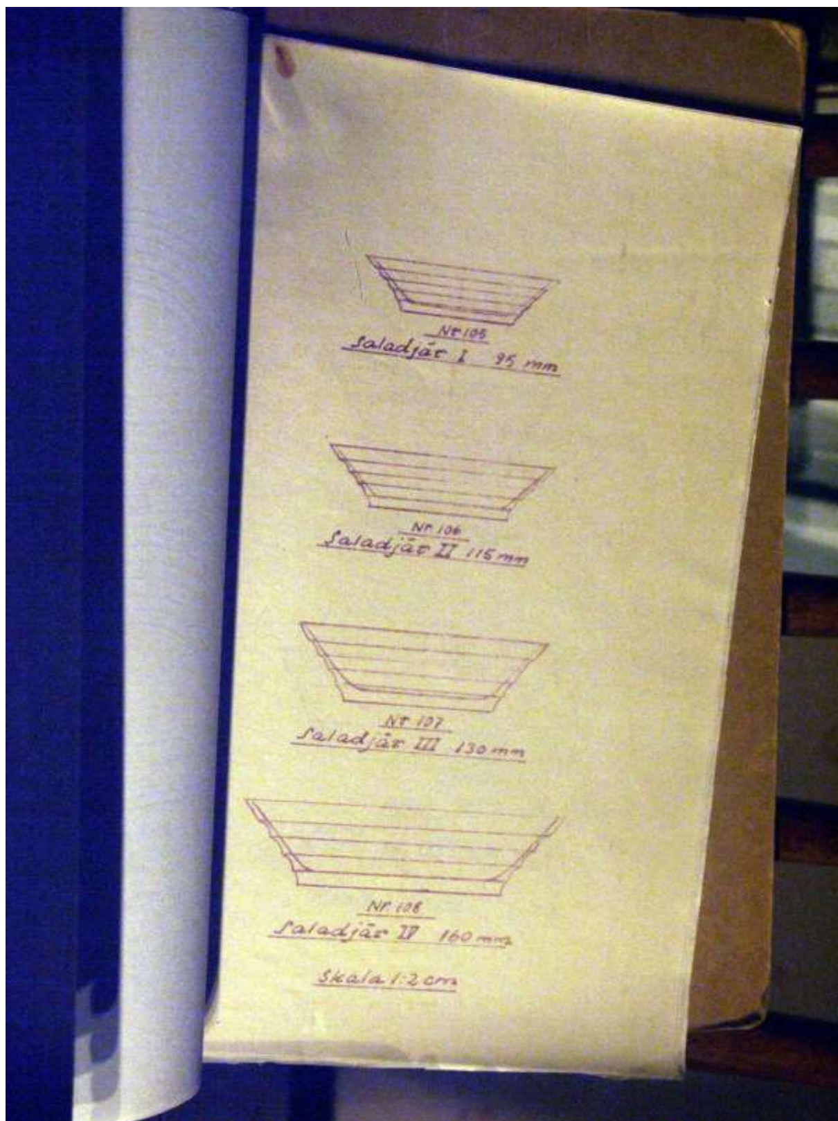
Nr 105 Saladjär I 95 mm Nr 106 Saladjär II 115 mm Nr 107 Saladjär III 130 mm Nr 108 Saladjär IV 160 mm Skala 1:2 cm
