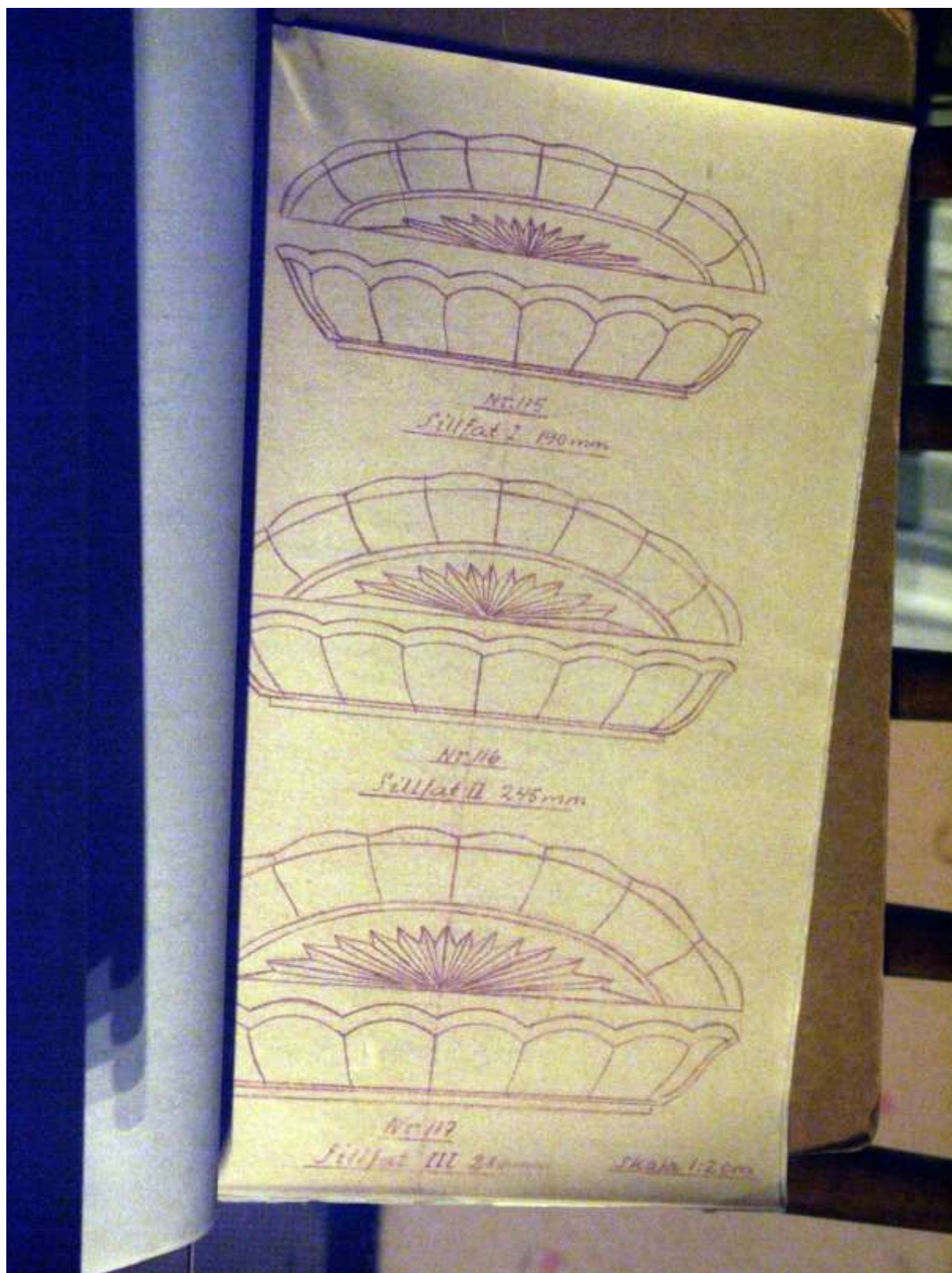
Nr 115 Sillfat I 140 mm Nr 116 Sillfat II 245 mm Nr 117 Sillfat III 280 mm Skala 1:2 cm
